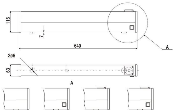
Двухполюсный выключатель
