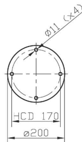
SH 480 D Монтажное основание
