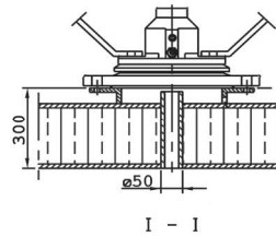
SH 480 BS Монтажное основание
