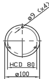
SH 480 BS Монтажное основание
