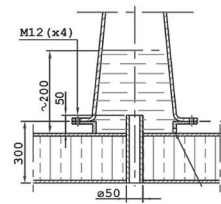
SH 480 BH Монтажное основание
