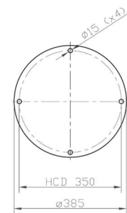
SH 480 DH Монтажное основание
