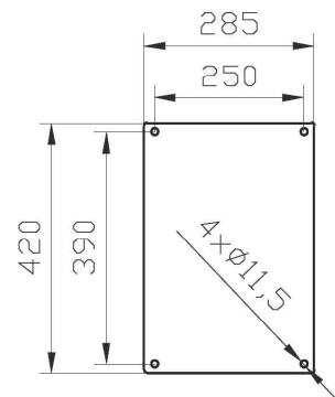
SH 480 R10 Монтажное основание
