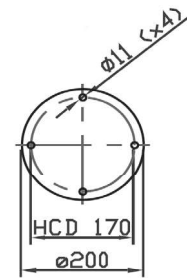
SH 480 BH Монтажное основание
